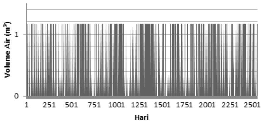
Gambar 5. Grafik Kebutuhan Air Harian yang Harus Dipenuhi dari Sumber Lain Tahun 2013-2018
