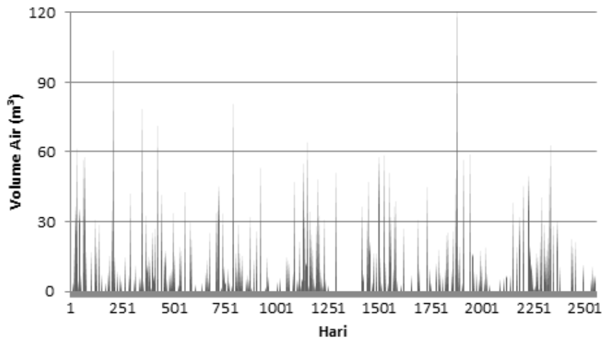
Gambar 4. Grafik Inflow Tahun Harian 2013-2018
