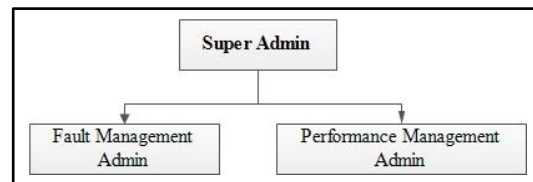
Gambar 8. Struktur User
